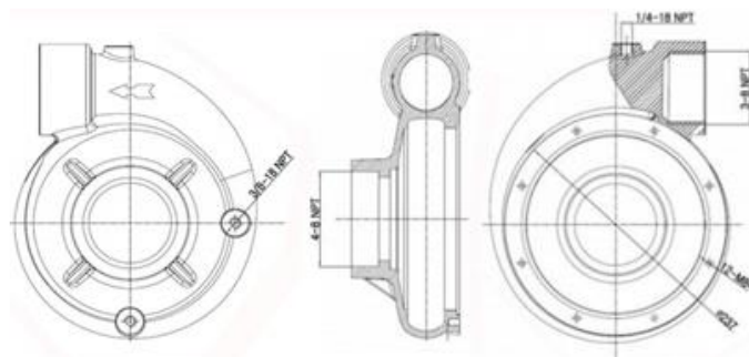
Tamaño del cuerpo de la bomba
